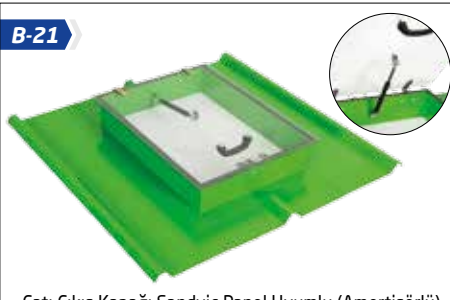
Çatı Çıkış Kapağı Sandviç Panel Uyumlu (Amortisörlü) Roof Exit Cover for Sandwich Panel (Shock absorber)
